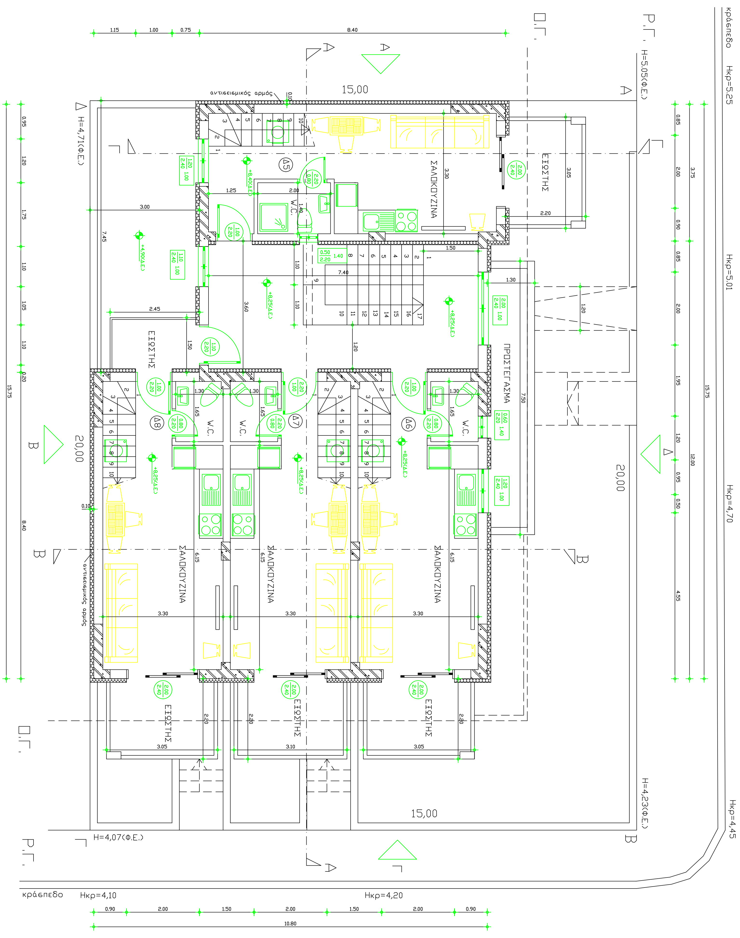
ΑΡΧΙΤΕΚΤΟΝΙΚΟ ΠΛΑΝΟ ΠΛΑΤΟΥΣ 10Μ.
